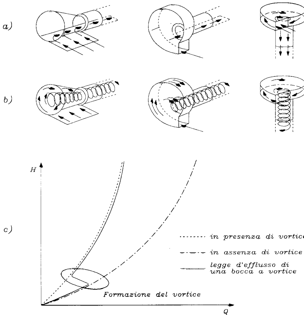
Figura 45 - Regolatori di portata a vortice
