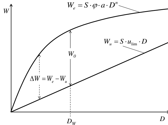
Figura 4 – Individuazione con il metodo delle sole piogge dell'evento critico D_w e del corrispondente volume critico W_o di laminazione, ovvero quello che massimizza il volume invasato.
