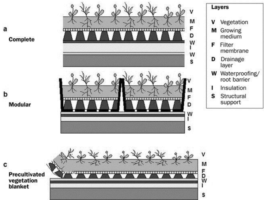
Figura 39 - Tecniche costruttive convenzionali di tetto verde estensivo (tratti dall'articolo Green Roofs as Urban Ecosystems: Ecological Structures, Functions, and Services, pubblicato sul sito http://www.bioone.org dell'American Institute of Biological Sciences). (a) Impianti completi: ogni componente, compresa la membrana del tetto, viene installato come parte integrante del tetto. (b) Impianti modulari: vassoi di vegetazione coltivata ex situ vengono installati al di sopra del sistema di copertura esistente. (c) strati di vegetazione precoltivata: il terreno di coltura, le piante, stuoie di drenaggio, e le barriere vengono srotolate sulla copertura esistente. Grafica: Jeremy Lundholm
