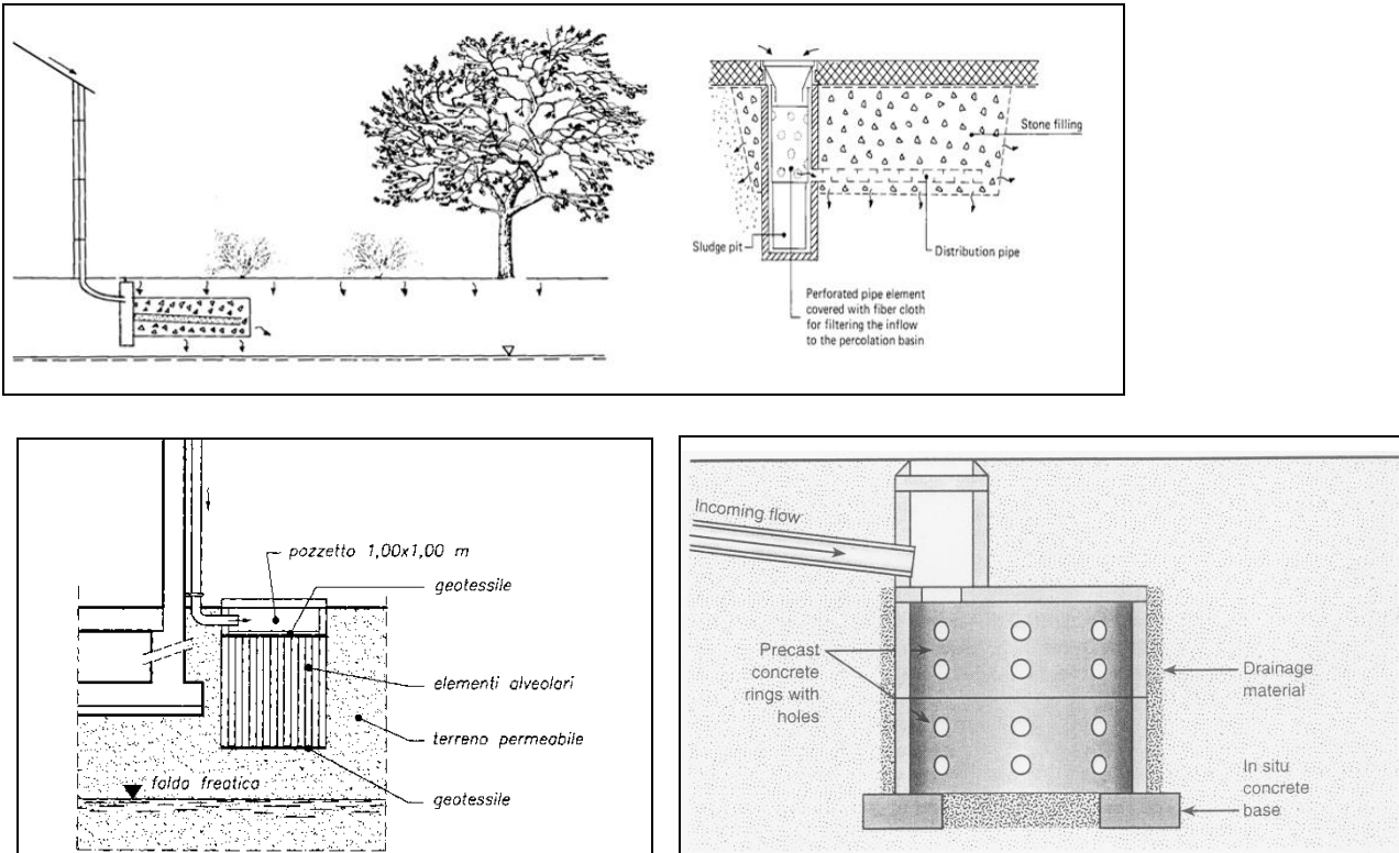
Figura 29 – Esempi di pozzi d’infiltrazione
