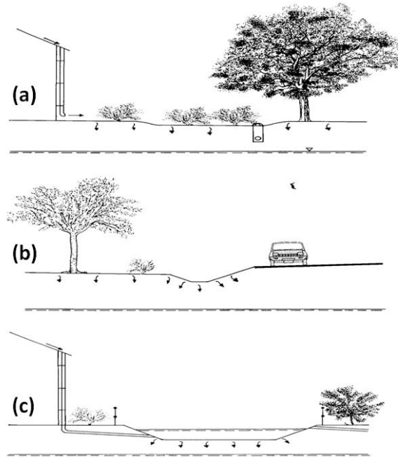
Figura 27 - Opere di infiltrazione [da: Urbonas e Stahre, 1993]
