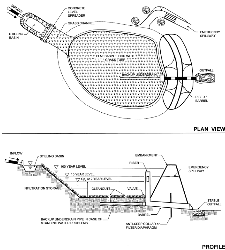
Figura 31 - Schema di un bacino di infiltrazione (Scheuler, 1992)
